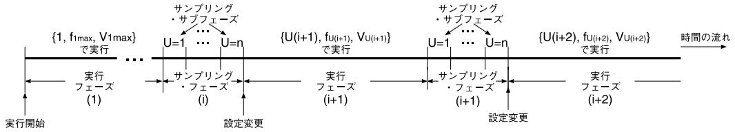
図 2 制御の概略
