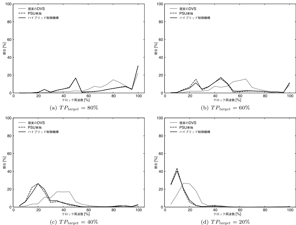
図 6 種々の TP_{target} に対する選択されたクロック周波数の分布
